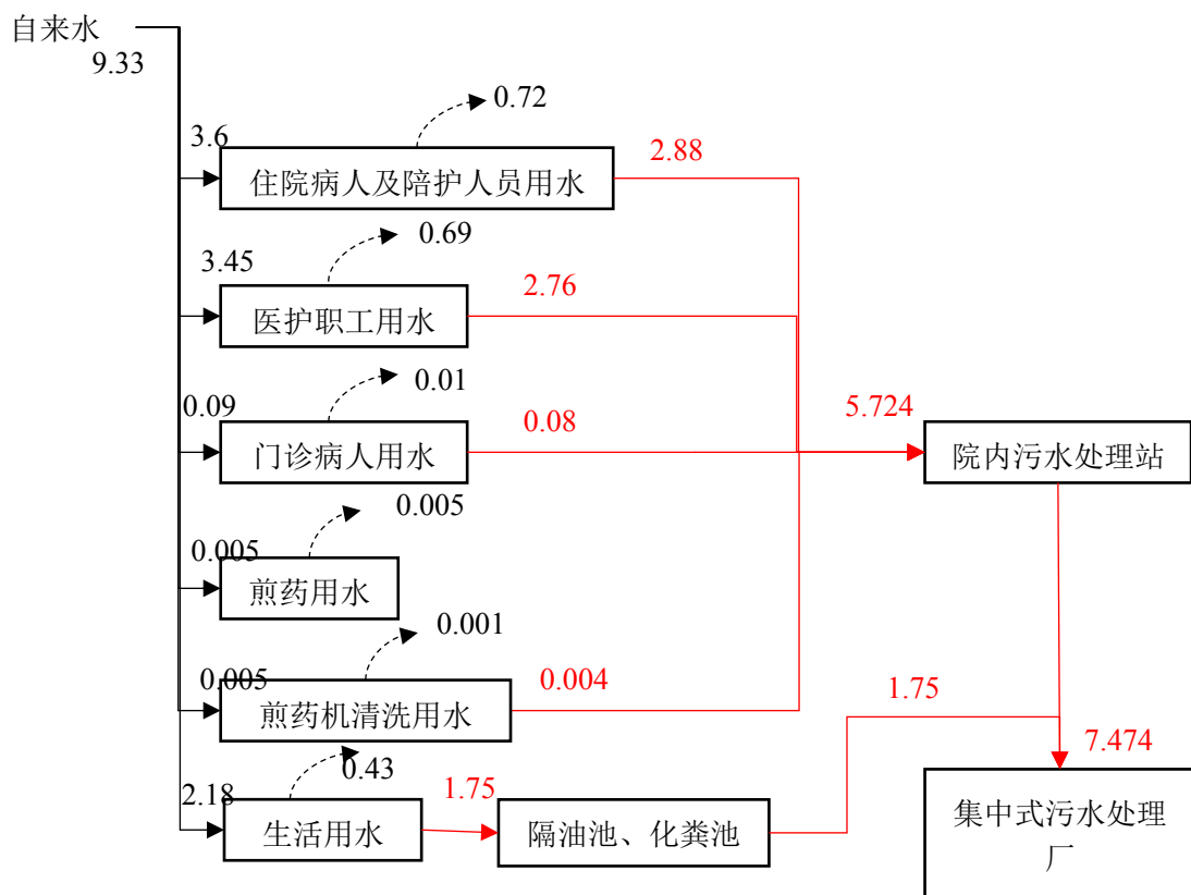
图 2-2 项目水量平衡图 单位:m³/d
